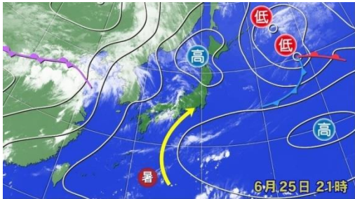
図1 地上天気図(6月25日21時の予想)
